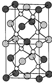
Chalcopyrite, E1 1 CuFeS 2
