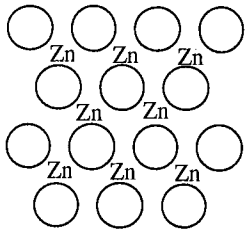
ZnO
